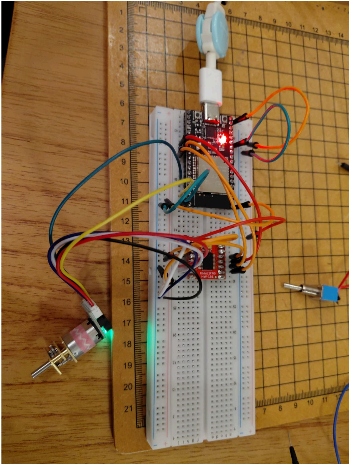
Figura 1 - Montagem da ponte H, motores e encoders.
